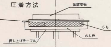
圧着方法
