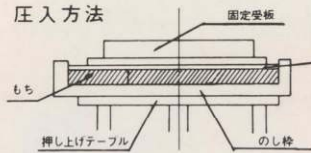
圧入方法
